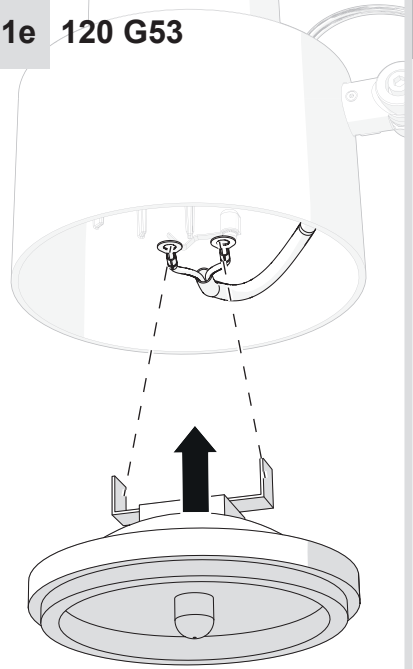
13e 120 G53
