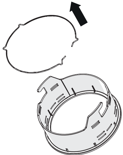
13e 120 G53
