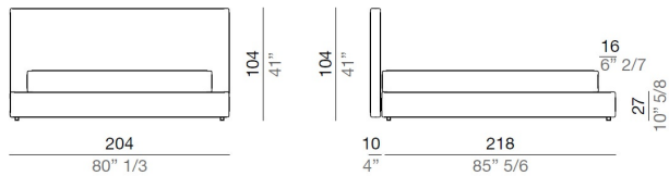
Double Bed 204 cm, base 172x202 cm - L204
